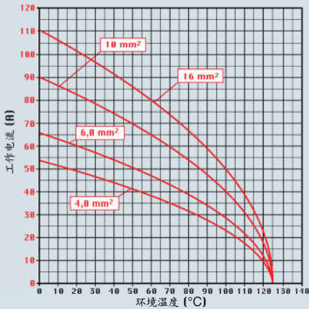
图表 CX 4/2 针
