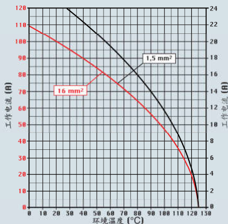
图表 CX 4/2 针
