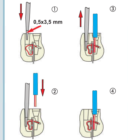
弹片端子连接
