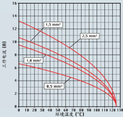
图表 CDD 76 针
